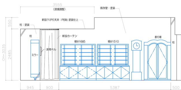
A面展開図
