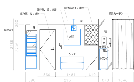
D面展開図
