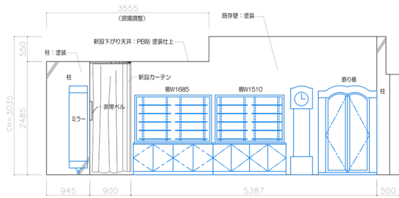
A面展開図
