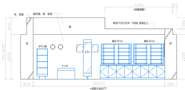
C面展開図
