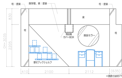
B面展開図
